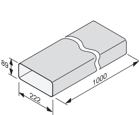
DFK-R 1000 • Lige stykke, 1 m M.-nr. 10811340 Pris kr. 275,00
