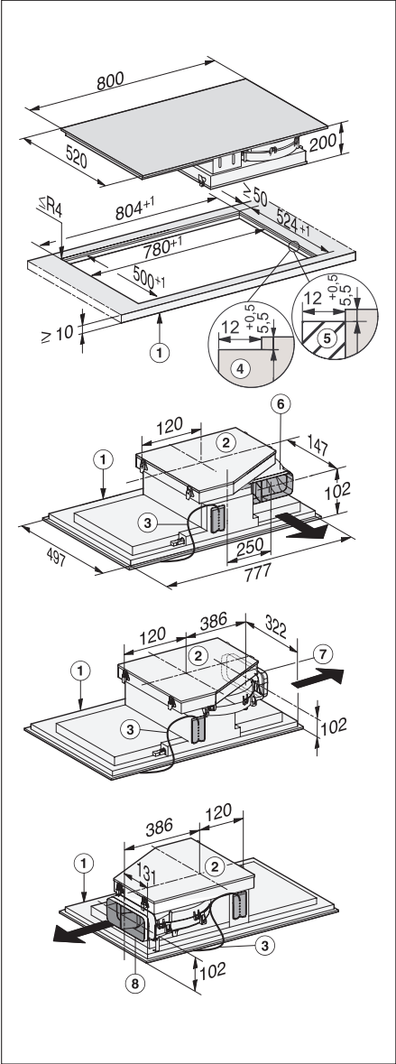
KMDA 7634 FL – Planforsænket
