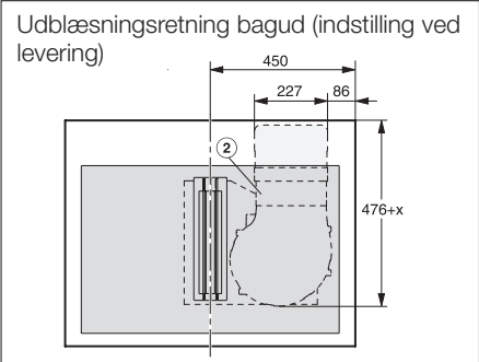
KMDA 7634 FR - Med stålramme, monteret oven på >600 mm dyb bordplade
