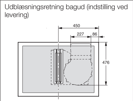
KMDA 7634 FL – Uden stålramme, planforsænket i 600 mm dyb bordplade
