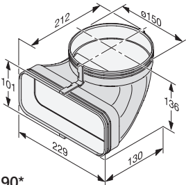
DFK-AK 90° • Adapter flad – rund 90° M.-nr. 11590720 Pris kr. 275,00
