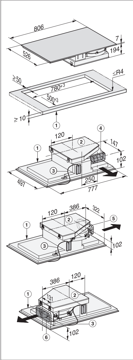
KMDA 7634 FR – Monteret på bordplade
