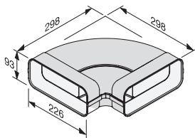
DFK-BH 90 • Horizontal bue 90° M.-nr. 10811390 Pris kr. 275,00
