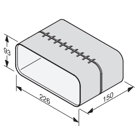
DFK-L • Ved pladsmangel (hvor DFK-V ikke kan bruges) • Ved montering sættes forlængerstykket DFK-L på fladkanalstykket, fladkanalen monteres, og forlængerstykket DFK-L skubbes over samlingen M.-nr. 11051270 Pris kr. 275,00
