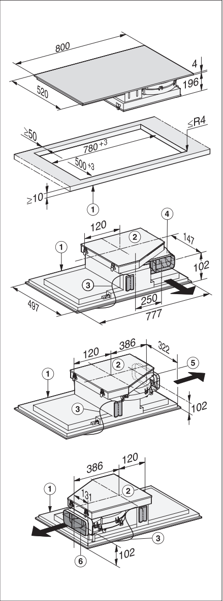
KMDA 7634 FL – Monteret på bordplade
