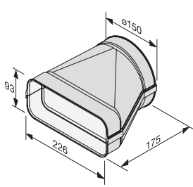
DFK-A • Adapter flad – rund M.-nr. 10811430 Pris kr. 275,00
