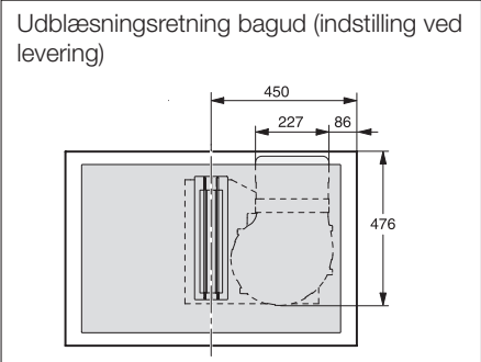
KMDA 7634 FL – Uden stålramme, monteret oven på 600 mm dyb bordplade
