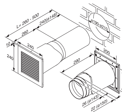
Aftræk til det fri DMK 150-1 • Murkasse M.-nr. 11258630 Pris kr. 1.495,00
